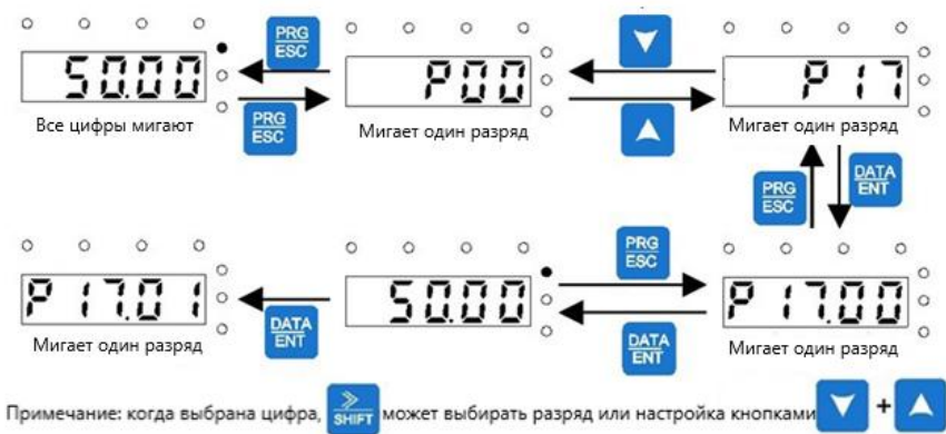
Рис. 5-5 Схема просмотра параметров состояния ПЧ
