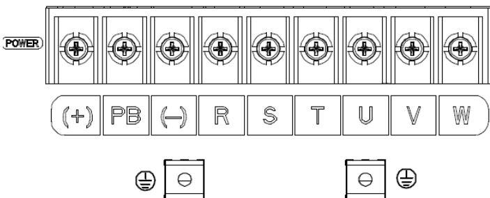
Рис. 4-11 Клеммы силовой цепи для моделей 7R5G/011P-015G/018P
