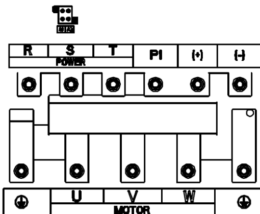
Рис. 4-16 Клеммы силовой цепи для моделей 132G/160P-200G/220P
