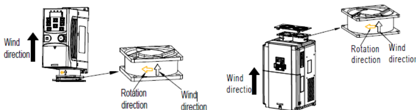
Рисунок 8-1 Диаграмма установки вентилятора
