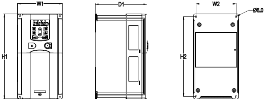
Рисунок В-3 Настенный монтаж для моделей 0R7G-15G/018P
