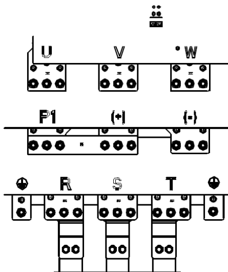
Рис. 4-18 Клеммы силовой цепи для моделей 355G/400P-500G
