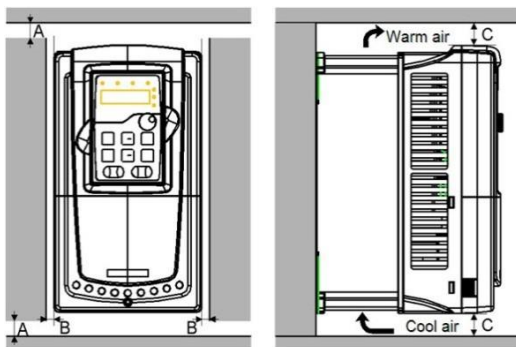
Рис. 4-3 Одиночная установка
