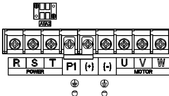
Рис. 4-14 Клеммы силовой цепи для моделей 037G/045P-055G/075P
