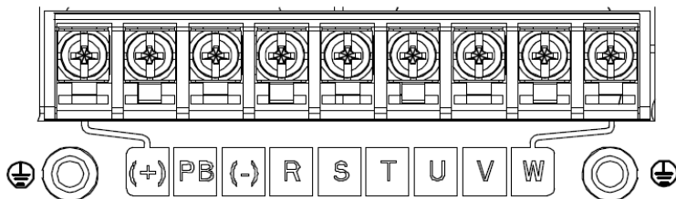
Рис. 4-10 Клеммы силовой цепи для моделей 0R7G-5R5G/7R5P
