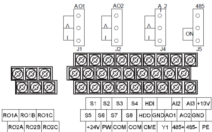
Рис. 4-21. Клеммы цепей управления моделей 015G/018P и ниже
