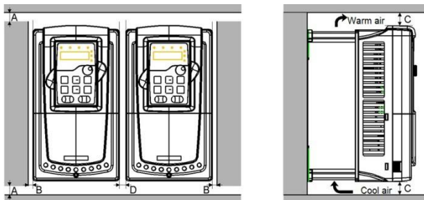
Рис. 4-4 Параллельная установка
