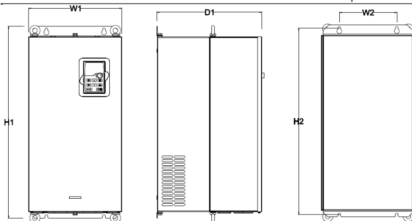
Рисунок В-5 Настенный монтаж для моделей 037G/045P-110G/132P
