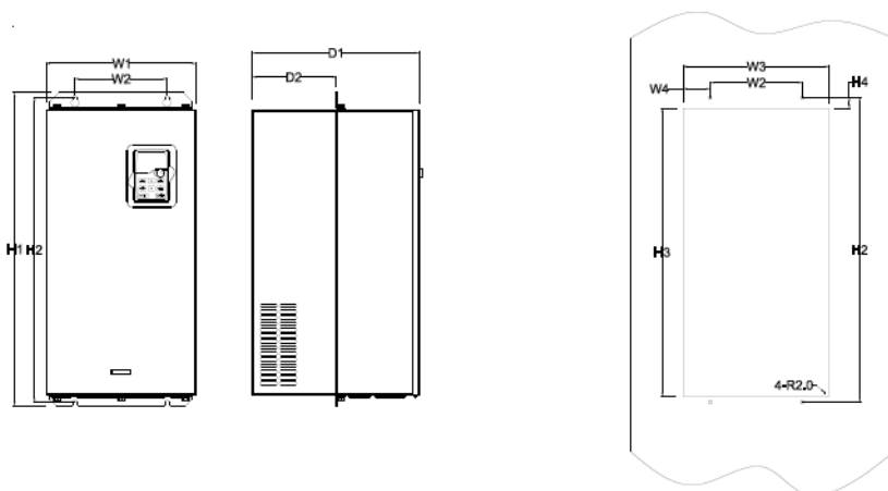
Рисунок В-10 Фланцевый монтаж для моделей 037G/045P-110G/132P
