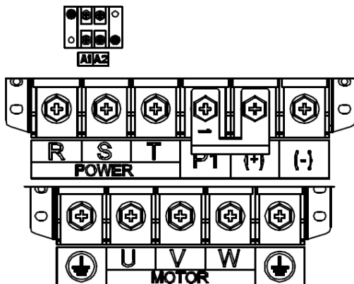
Рис. 4-15 Клеммы силовой цепи для моделей 075G/090P-110G/132P
