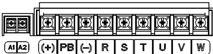
Рис. 4-12 Клеммы силовой цепи для моделей 018G/022P
