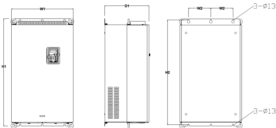
Рисунок В-6 Настенный монтаж для моделей 132G/160P-200G/220P
