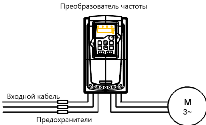
Рис. 4-24 Подключение предохранителей
