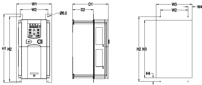
Рисунок В-8 Фланцевый монтаж для моделей 0R7G-015G/018P
