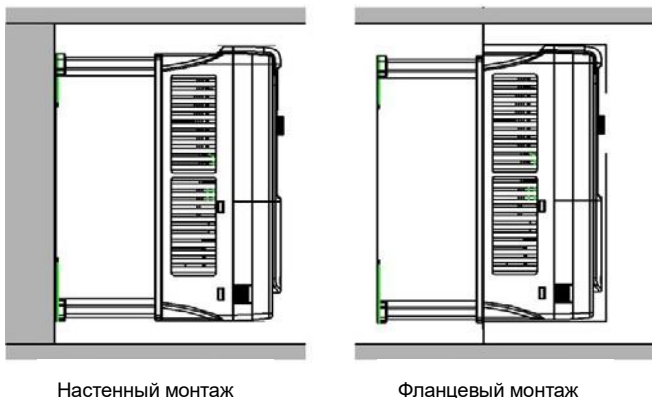
Рис. 4-2 Способы установки
