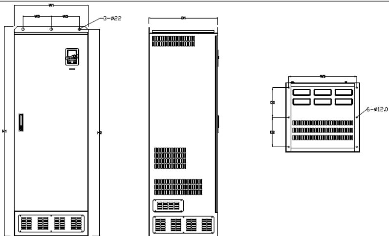
Рисунок В-13 Напольный монтаж для моделей 355G/400P-500G
