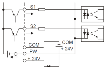
Внешнее питание (PNP режим)
