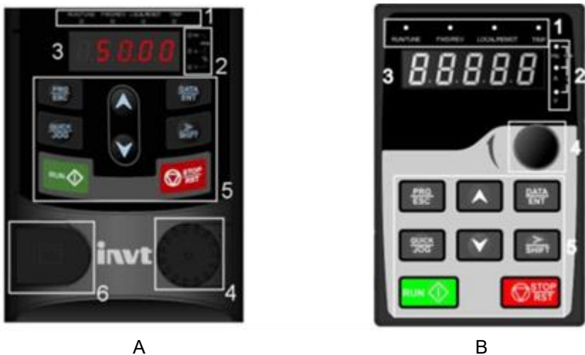
Рис. 5-1 Внешний вид панели управления
