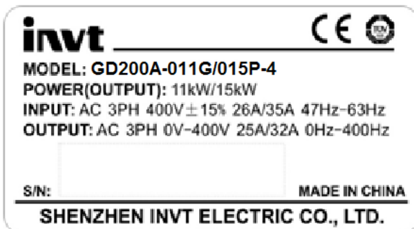
Рис. 3-3 Табличка ПЧ
