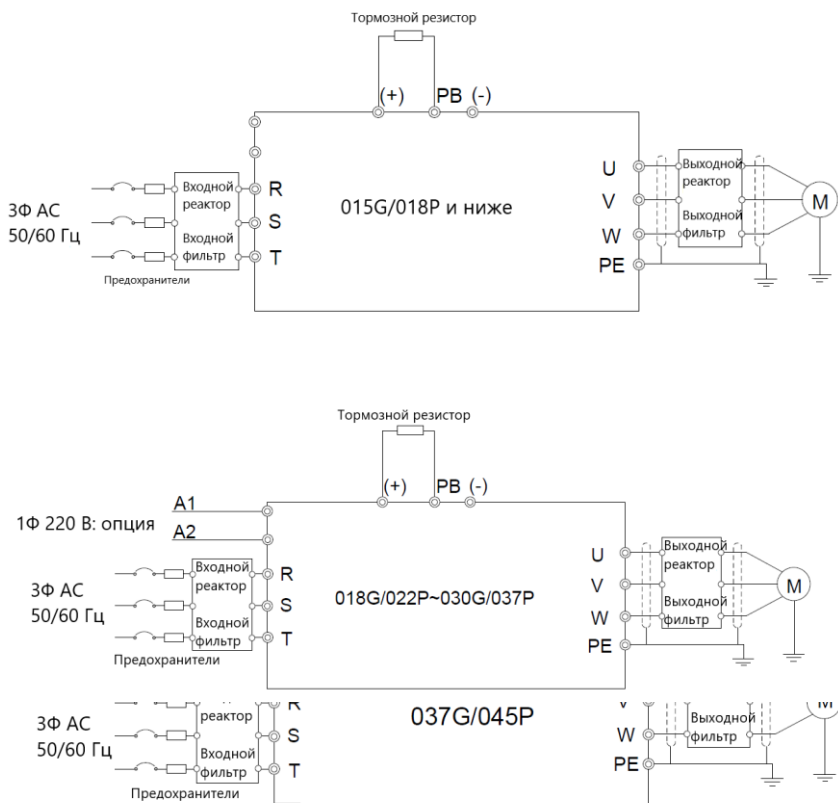
Рис. 4-9 Схема подключения силовых цепей для моделей 037G/045P и выше
