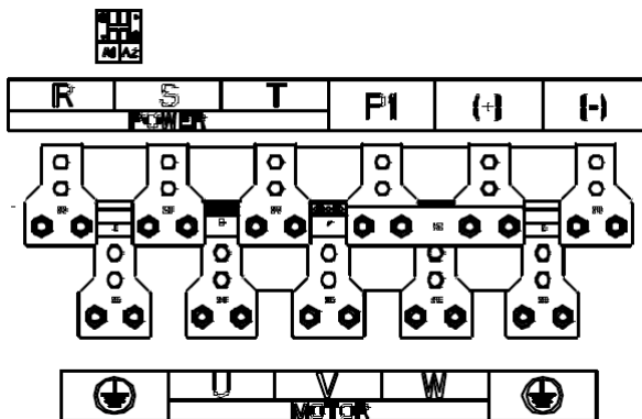
Рис. 4-17 Клеммы силовой цепи для моделей 220G/250P-315G/355P
