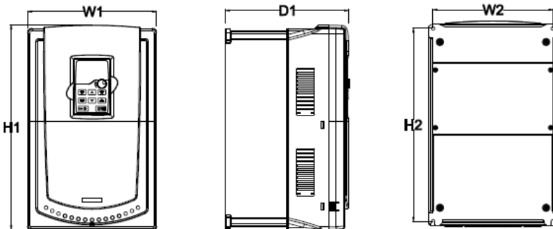
Рисунок В-4 Настенный монтаж для моделей 018G/022P-030G/037P
