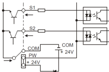
Внутреннее питание (NPN режим)
