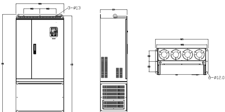
Рисунок В-12 Напольный монтаж для моделей 220G/250P-315G/355P
