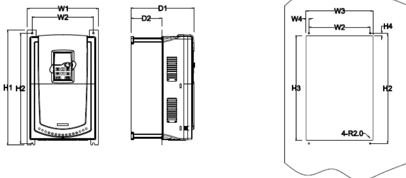
Рисунок В-9 Фланцевый монтаж для моделей 018G/022P-030G/037P
