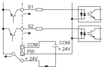
Внутреннее питание (PNP режим)
