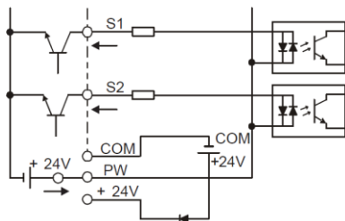
Внешнее питание (NPN режим)
