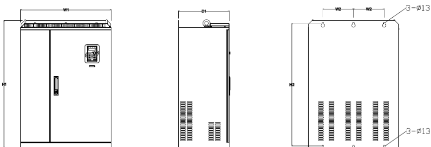
Рисунок В-7 Настенный монтаж для моделей 220G/250P-315G/355P
