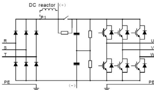
Рис. 3-2 Схема силовой цепи (модели 037G/045P и выше)
