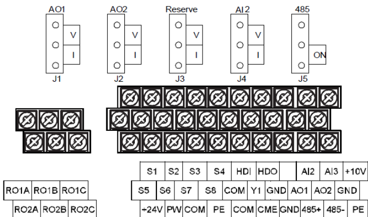
Рис. 4-22. Клеммы цепей управления моделей 018G/022P и выше
