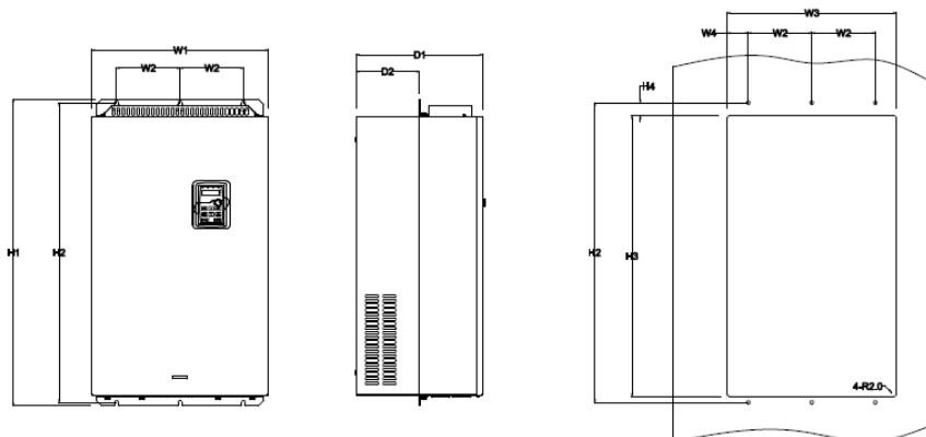
Рисунок В-11 Фланцевый монтаж для моделей 132G/160P-200G/220P
