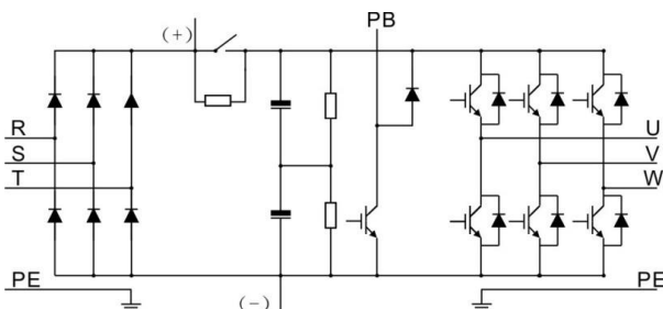
Рис. 3-1 Схема силовой цепи (модели 030G/037P и ниже)
