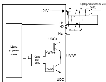
Рисунок Е-2 Схема подключения функции STO
