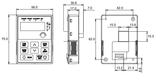
Рисунок D-5 Отверстия для крепления панели без кронштейна
