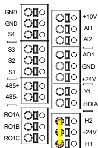
Рисунок Е-1 Перемычка между +24V на H1 и H2
