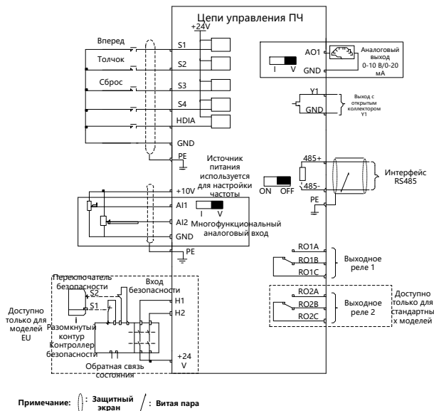
Рисунок 4-9 Схема цепей управления
