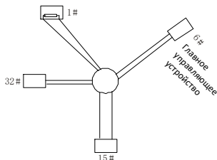
Рисунок 7-3 Соединение в звезду
