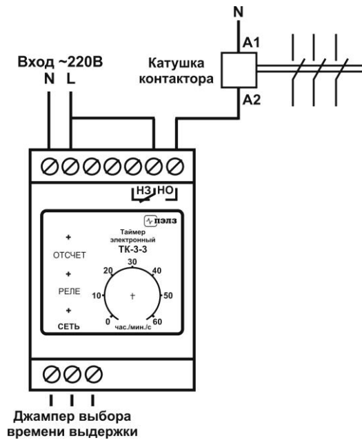
Рис. 1. Расположение контактов на клеммниках реле времени и вариант подключения к катушке контактора.
