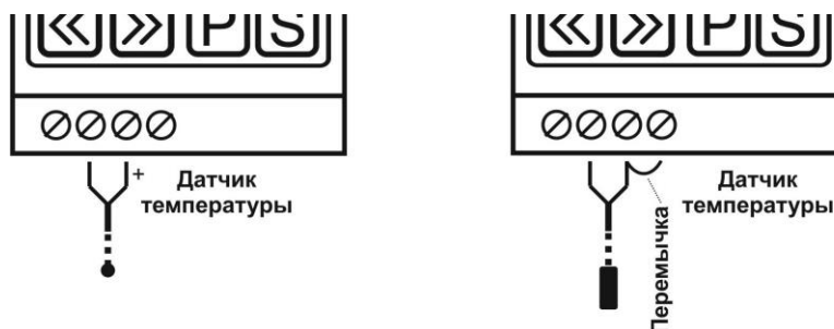
Рис 1. Варианты подключения датчика температуры.
