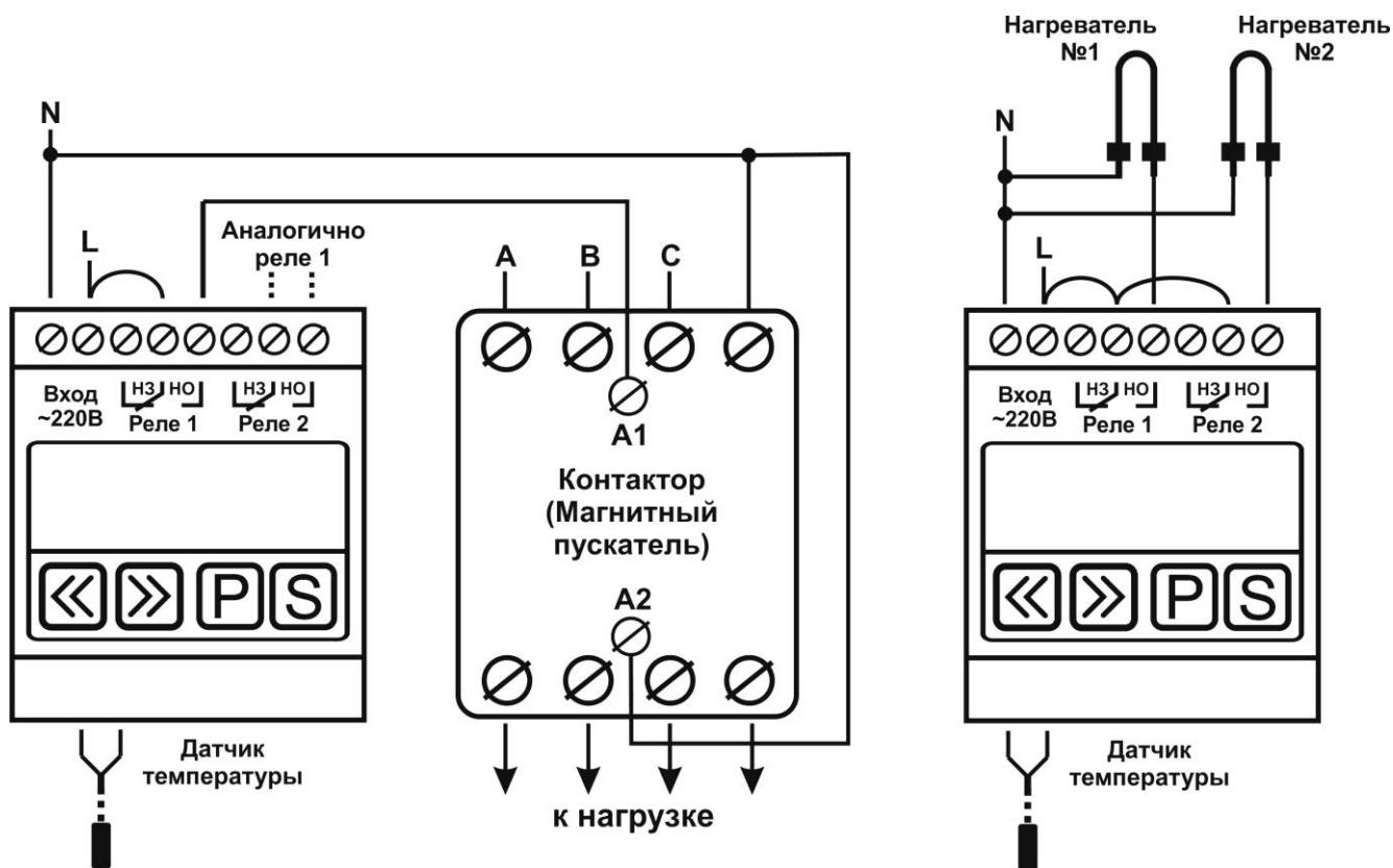
Рис 2. Слева: Вариант подключения нагрузки на 380В через контактор с катушкой на 220В. Справа: Вариант подключения нагрузки на 220В напрямую к МПРТ-112Т.
