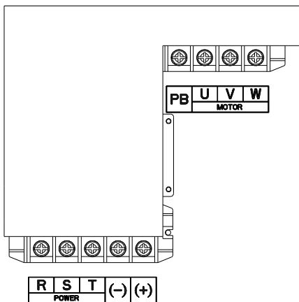
Рис 4. Силовые клеммы 045G/055P–055G/075P
