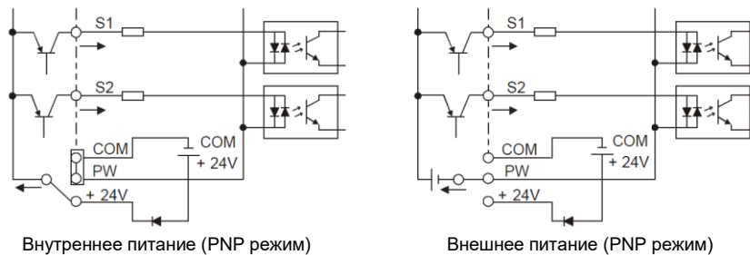
Рис 4.18 PNP режим
