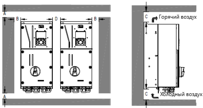
Рис 4.4 Параллельная установка
