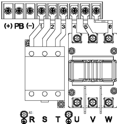
Рис 4.9 Силовые клеммы 7R5G/011P–015G/018P
