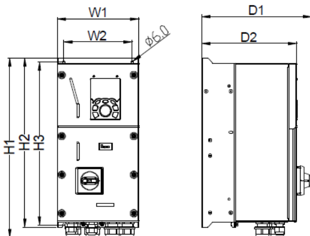
Рис С.1 Схема настенного монтажа ПЧ моделей 004G/5R5P–037G/045P
