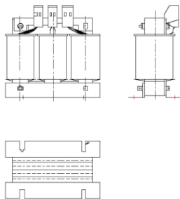
Входной реактор
