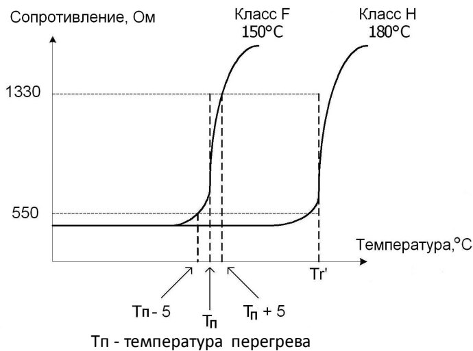
Характеристика (а) и подключение (б) термистора.
