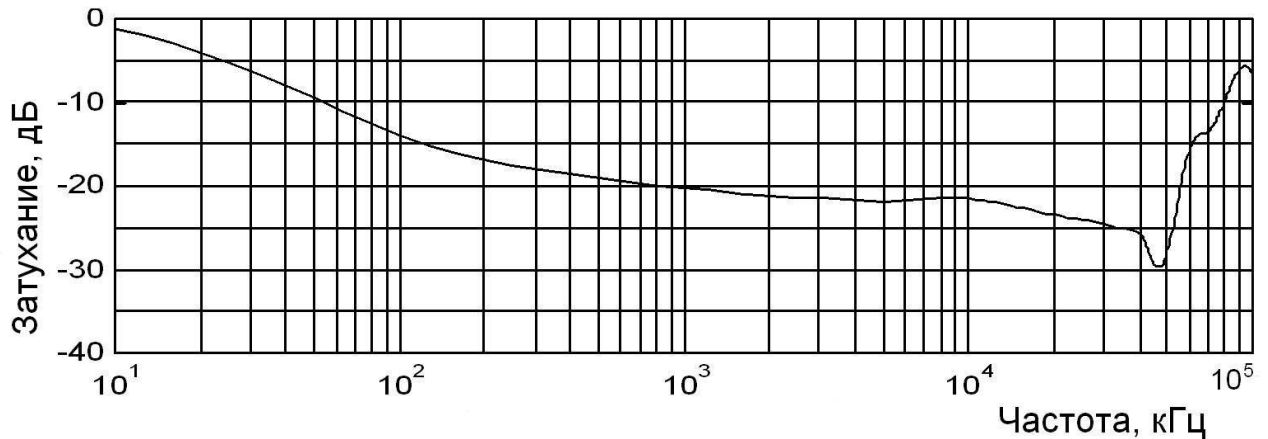
Характеристика затухания (пример для 10 витков провода)
